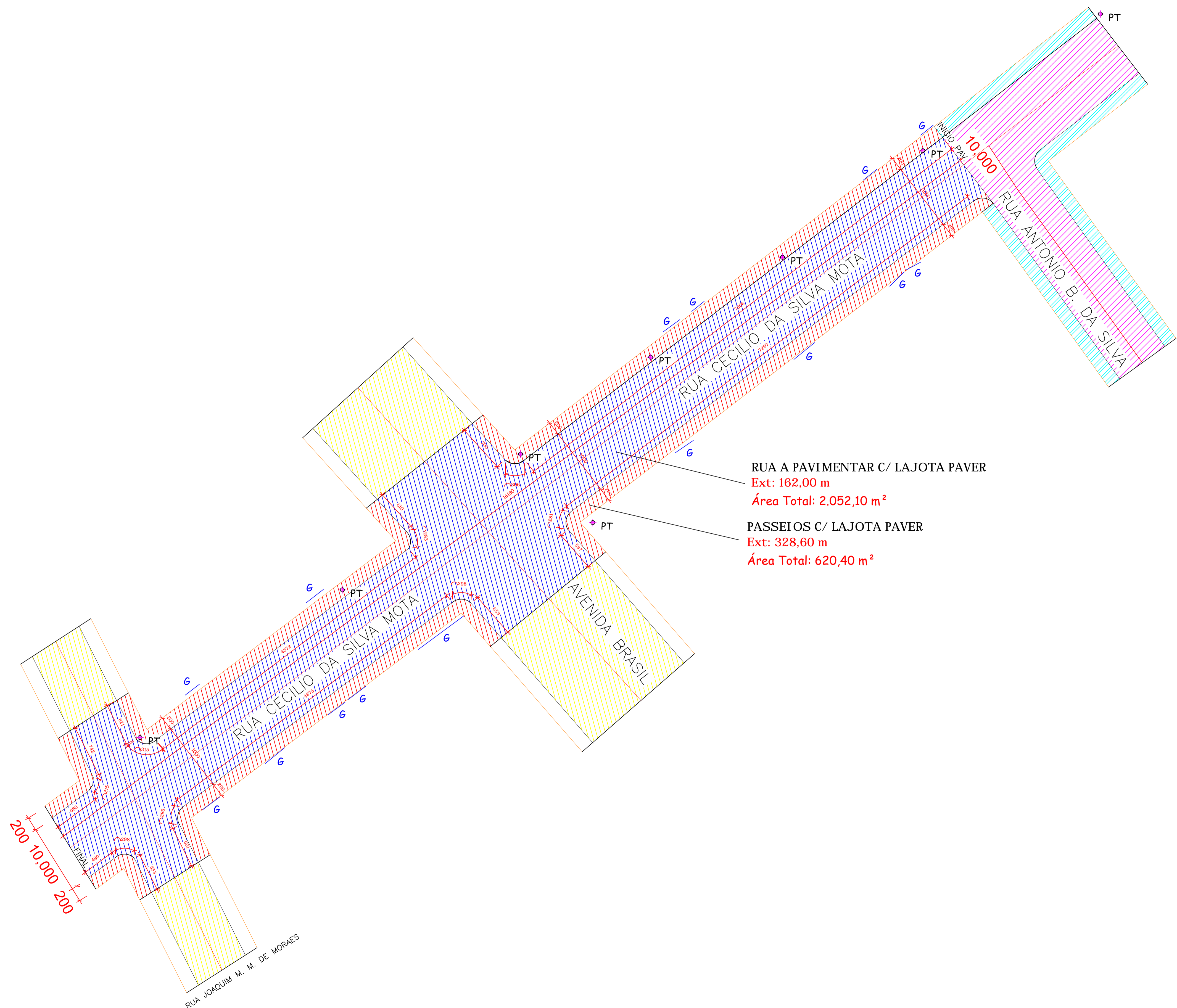
PROJETO LAYOUT Escala 1/300
