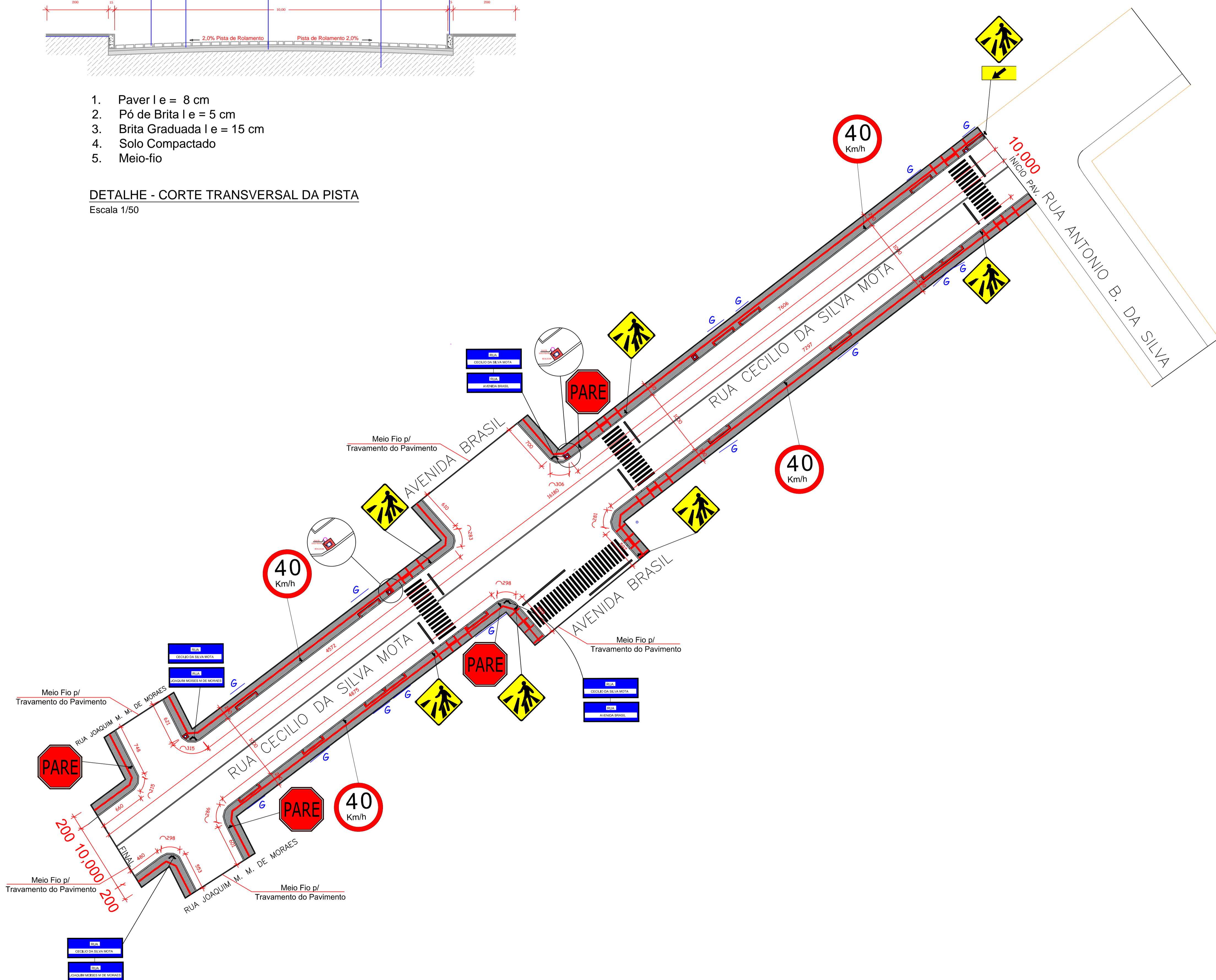
PROJETO DE SINALIZAÇÃO VERTICAL E HORIZONTAL Escala 1/50
