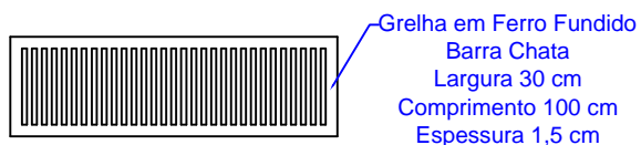
Detalhe 01 - Grelha Escala 1:25
