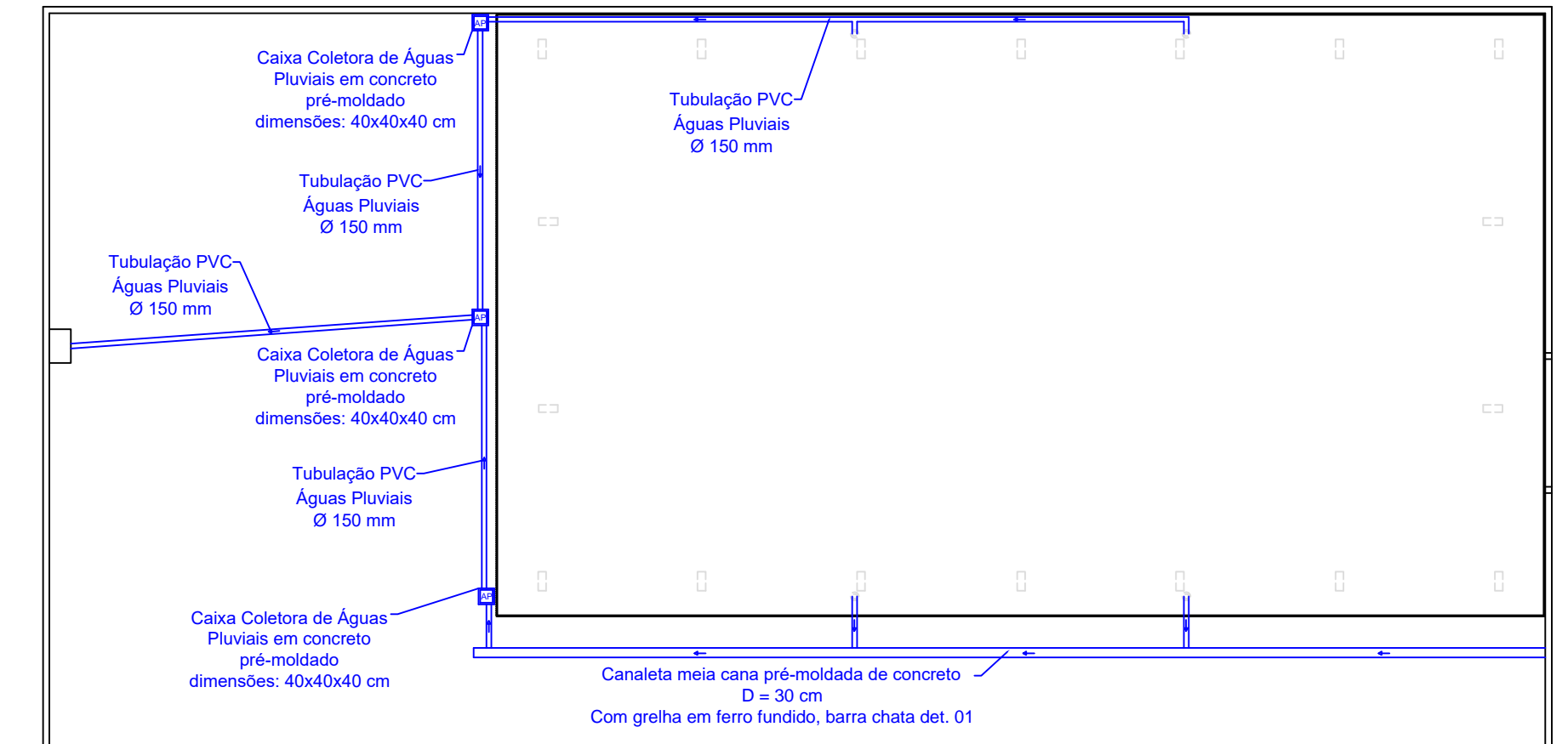
Disposição de Águas Pluviais Escala 1:200
