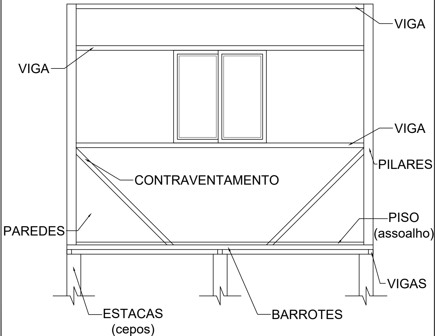
DETALHE ESTRUTURAL 02: Disposição de Elementos de Infraestrutura e Superestrutura Escala 1:25
