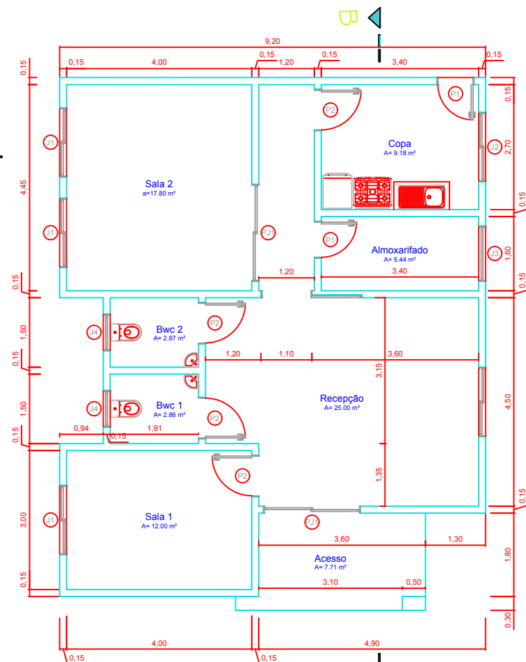
Planta Baixa Esc 1/50
