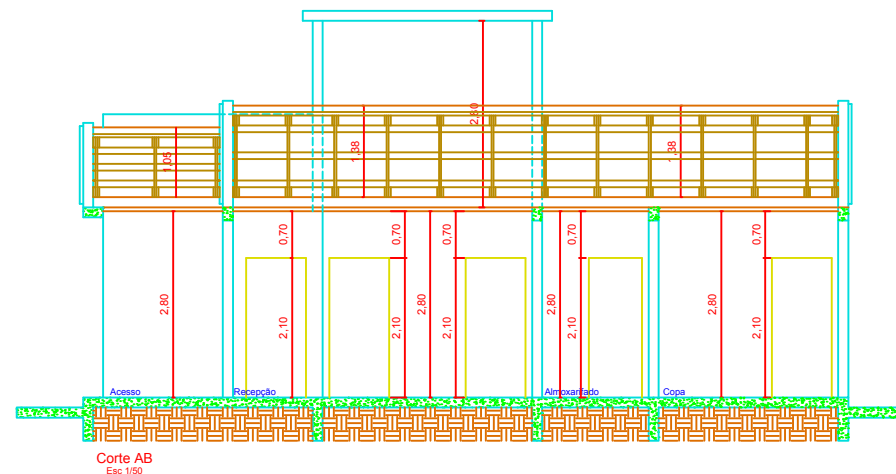
Corte AB Esc 1/50
