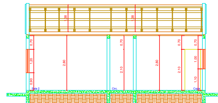
Corte CD Esc 1/50
