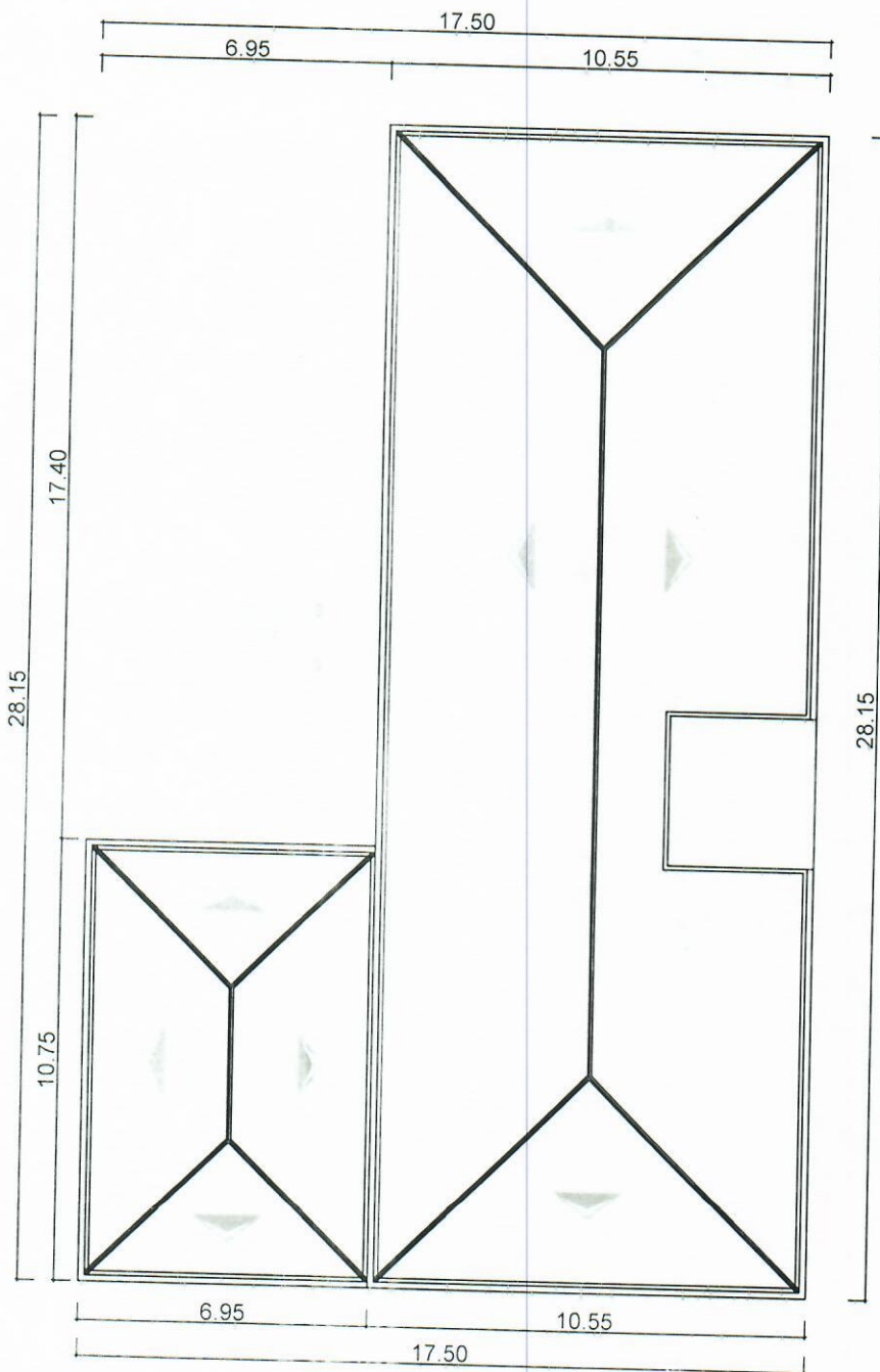
PLANTA DE COBERTURA Escala 1:200 A = 371,70 m 2
