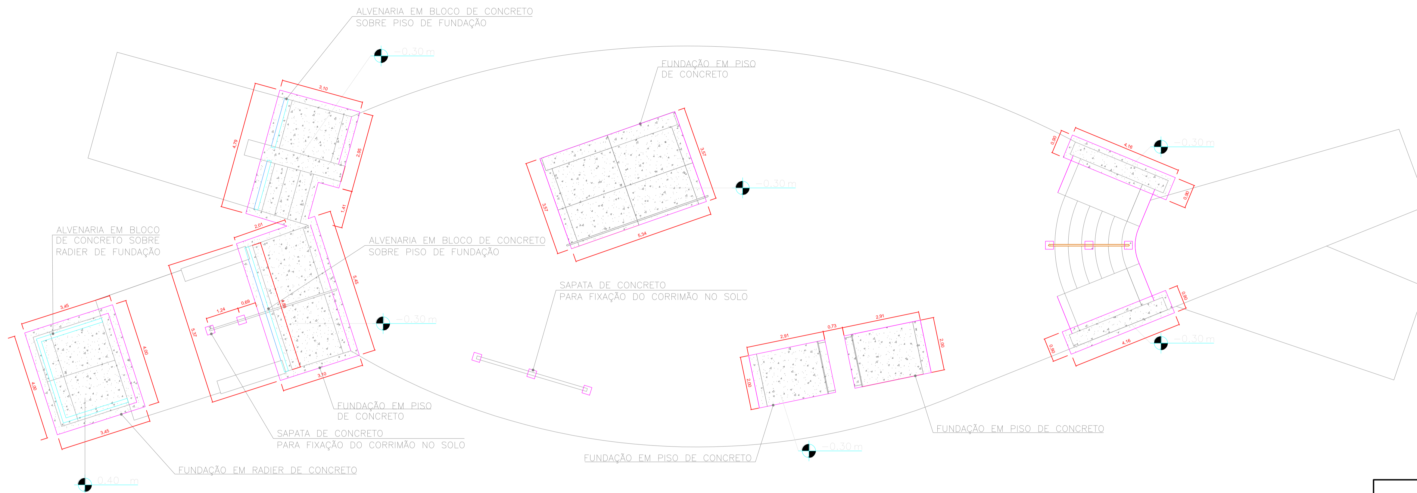
PLANTA BAIXA ALVENARIA E PISO PISTA DE SKATE Área Total: 517,80m 2 Escala 1/50
