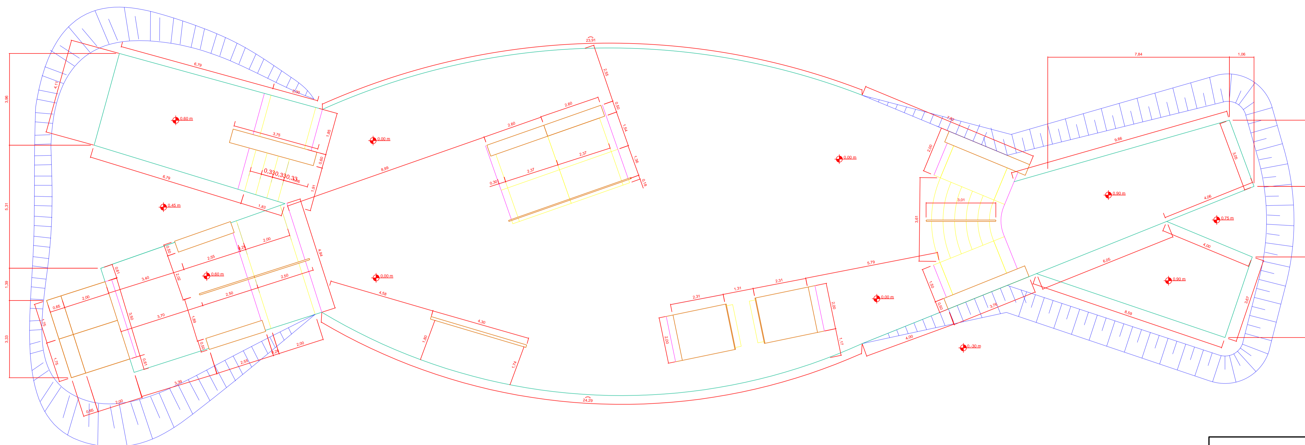
PLANTA BAIXA TÉCNICA E NIVEIS PISTA DE SKATE Área Total: 517,80m 2 Escala 1/50
