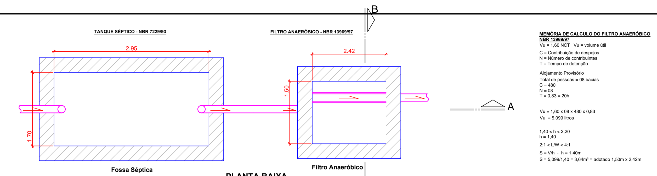
PLANTA BAIXA Sem Escala
