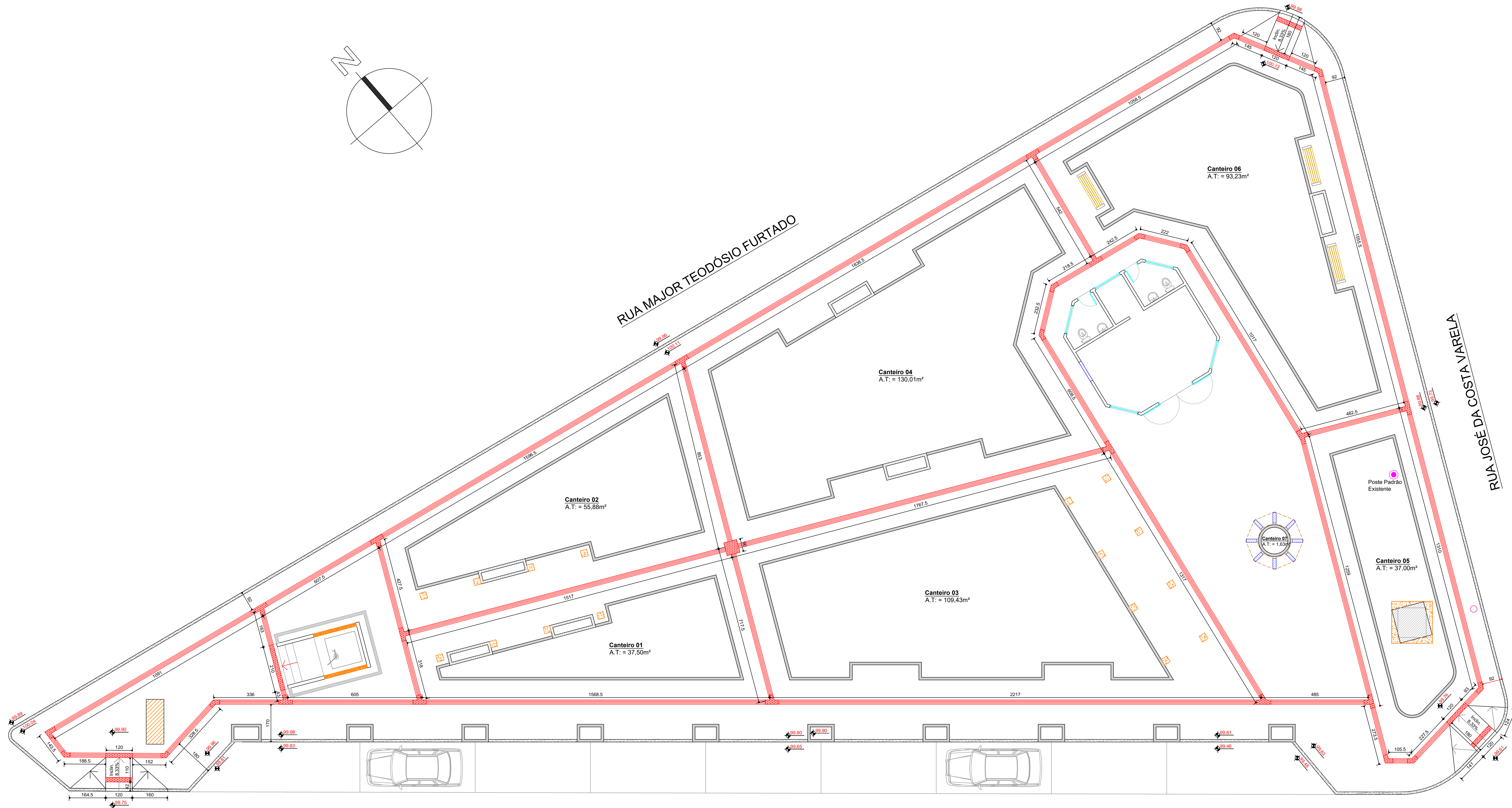
PLANTA BAIXA - Acessibilidade Escala 1/75
