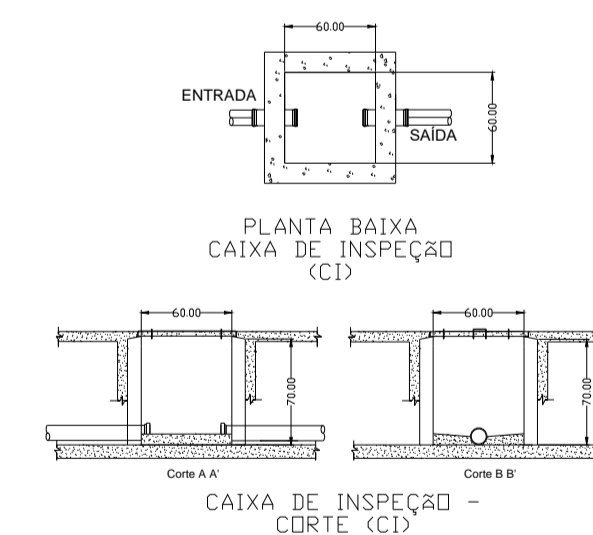
CAIXA DE INSPEÇÃO ESC: 1/25
