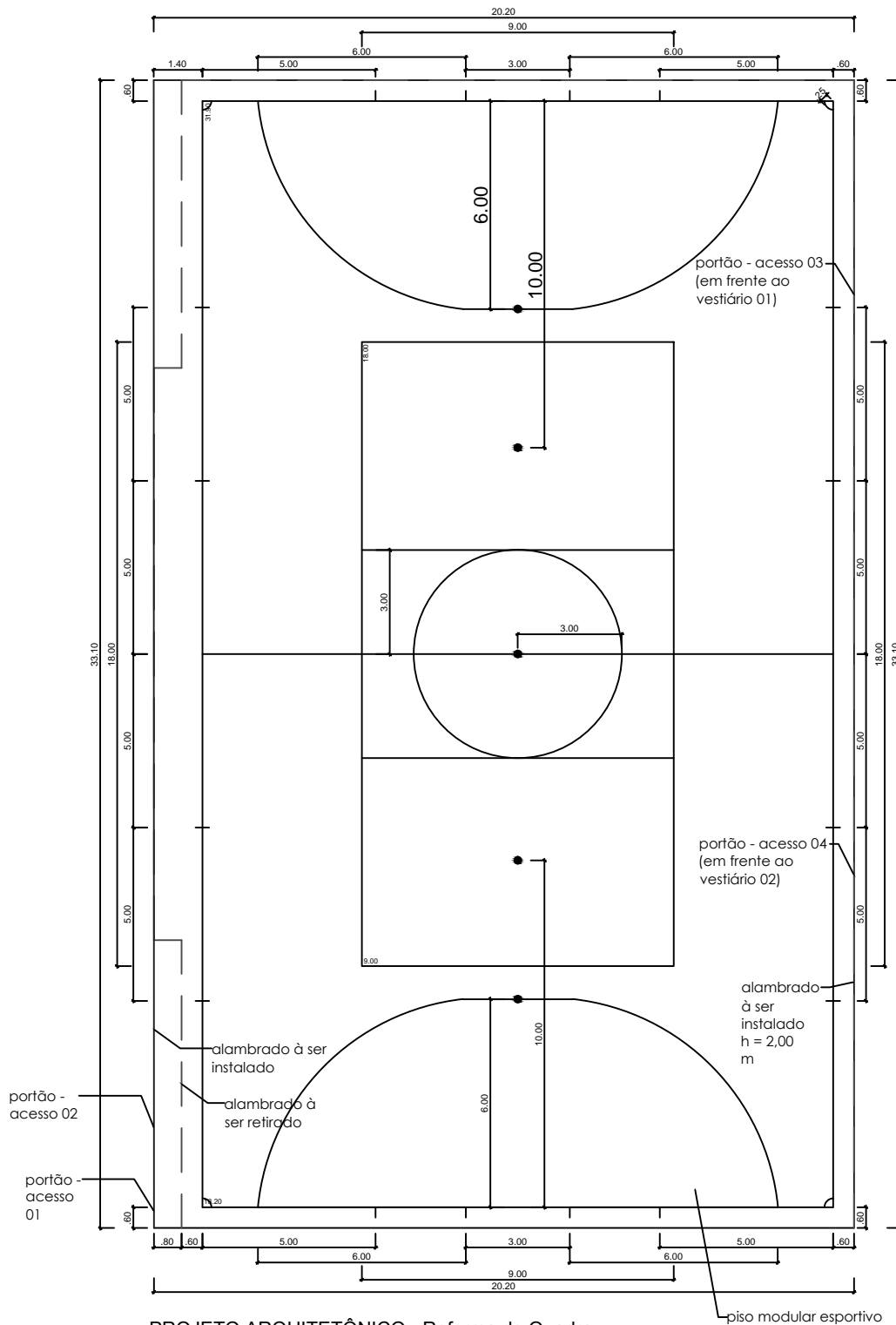
PROJETO ARQUITETÔNICO - Reforma de Quadra Escala 1:200 Área: 668,62 m 2
