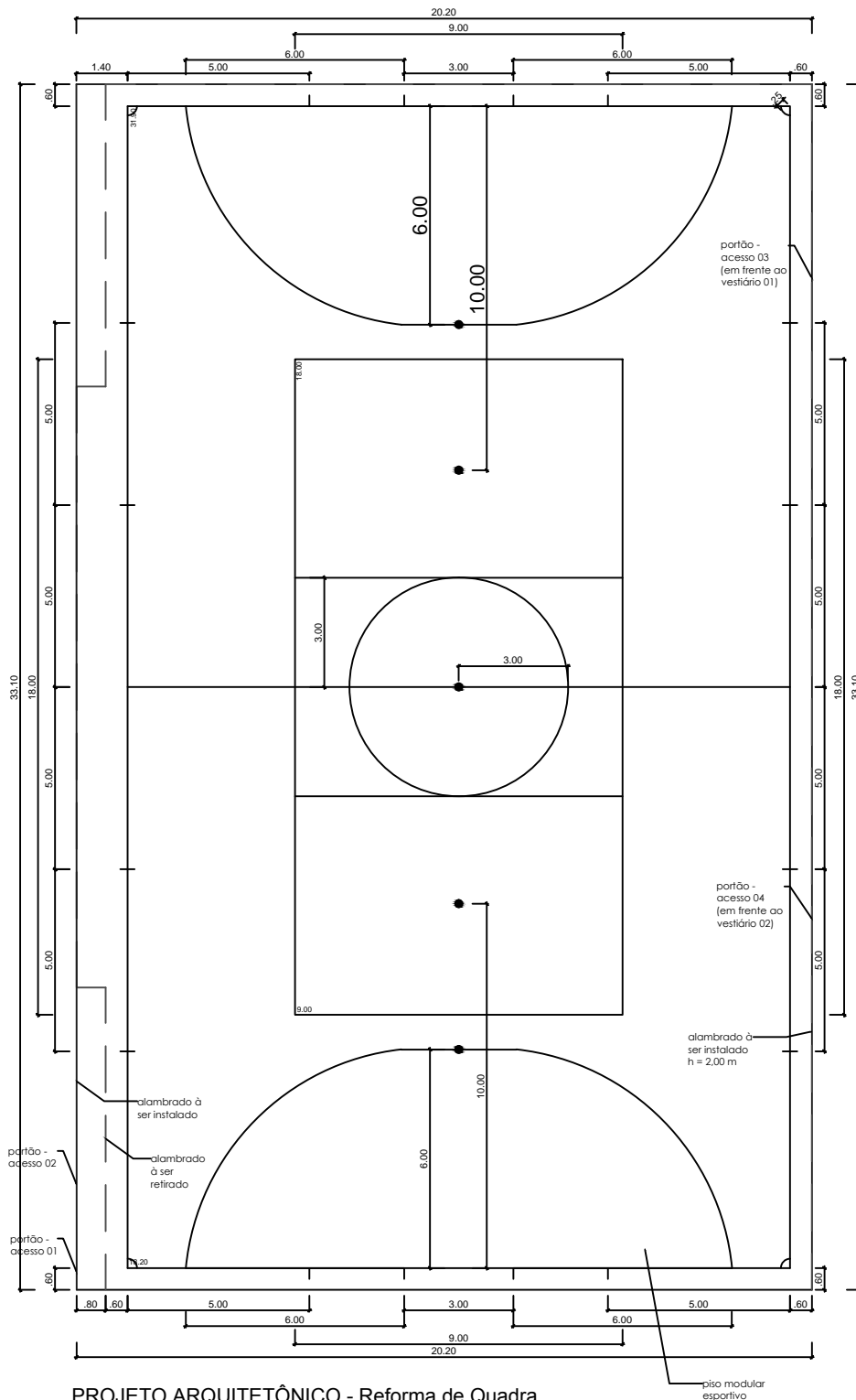
PROJETO ARQUITETÔNICO - Reforma de Quadra Escala 1:200 Área: 668,62 m 2
