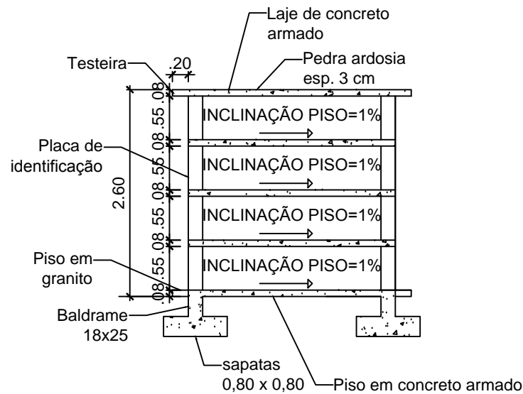
CORTE BB' Escala 1:75
